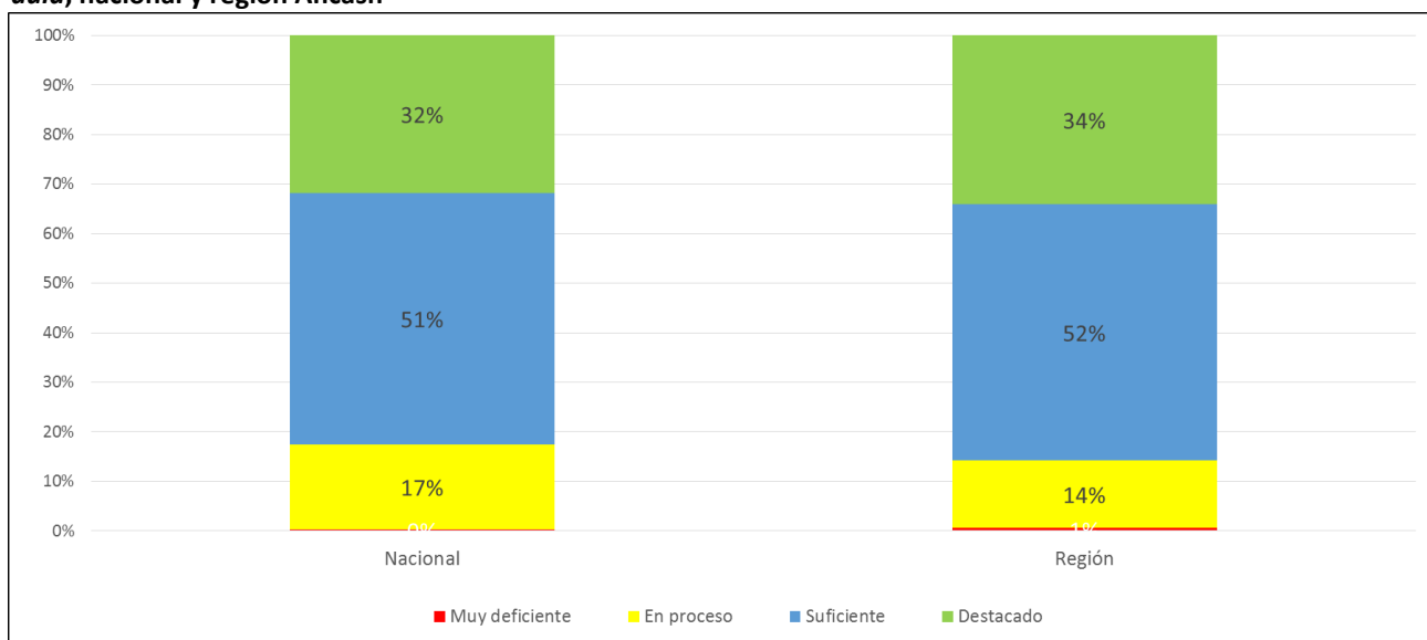
Gráfico 8
