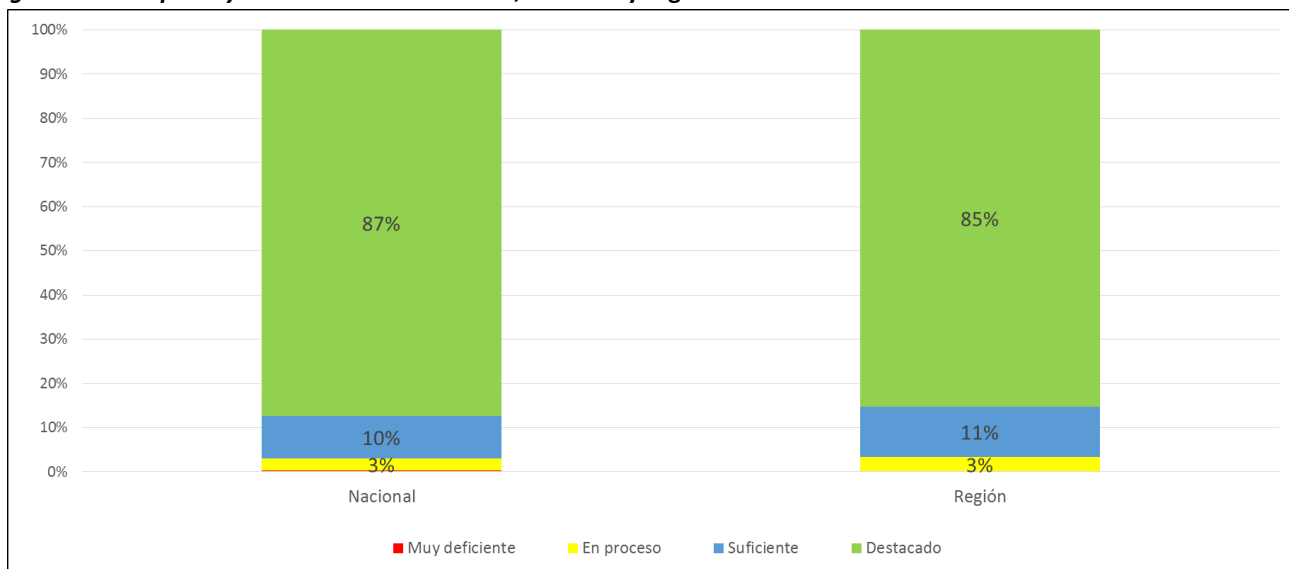
Gráfico 11
