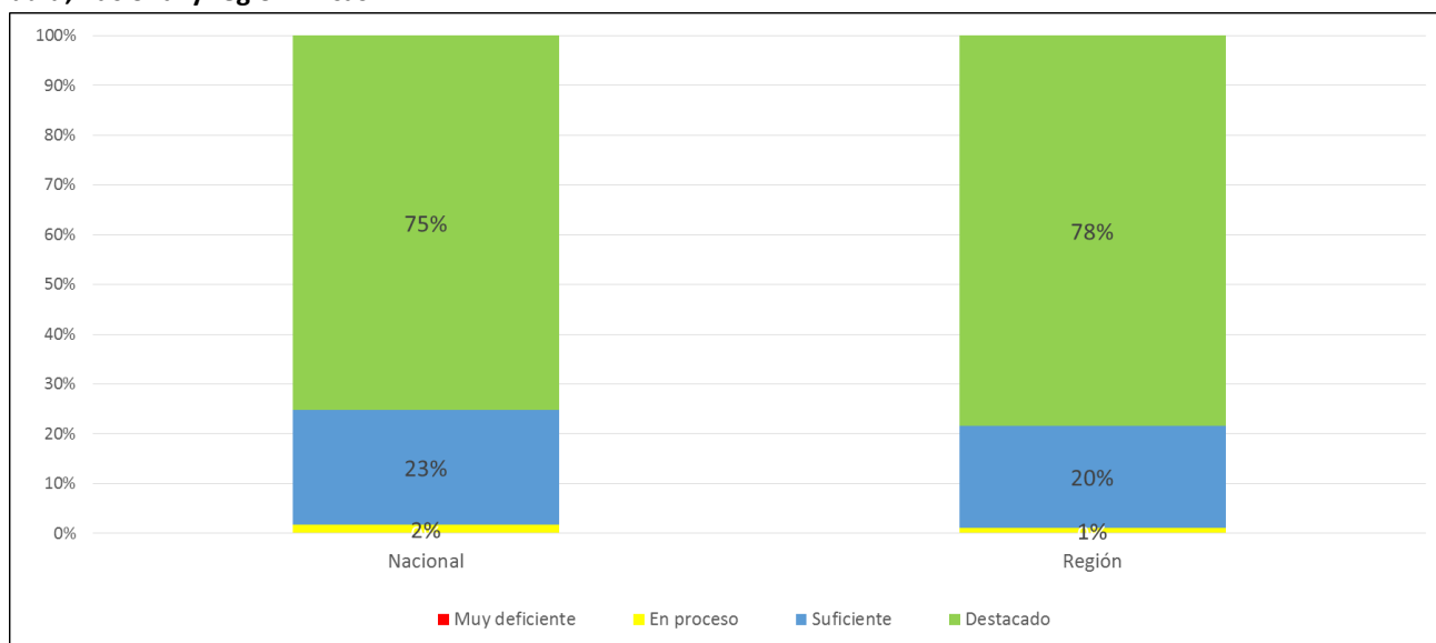
Gráfico 6
