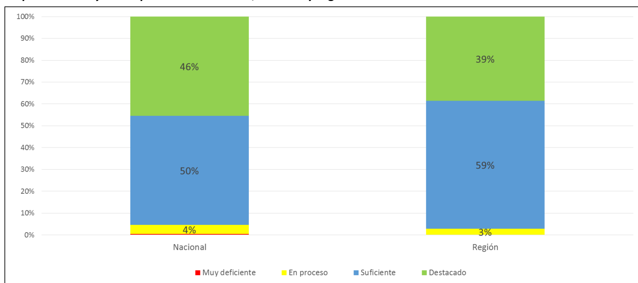
Gráfico 16
