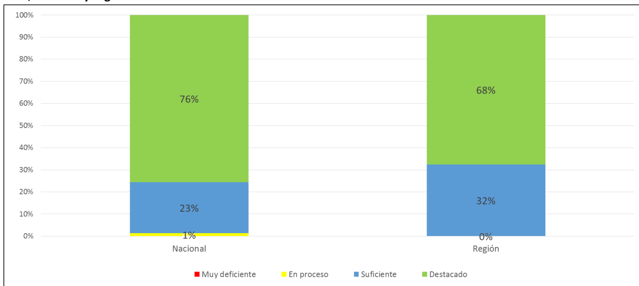
Gráfico 9
