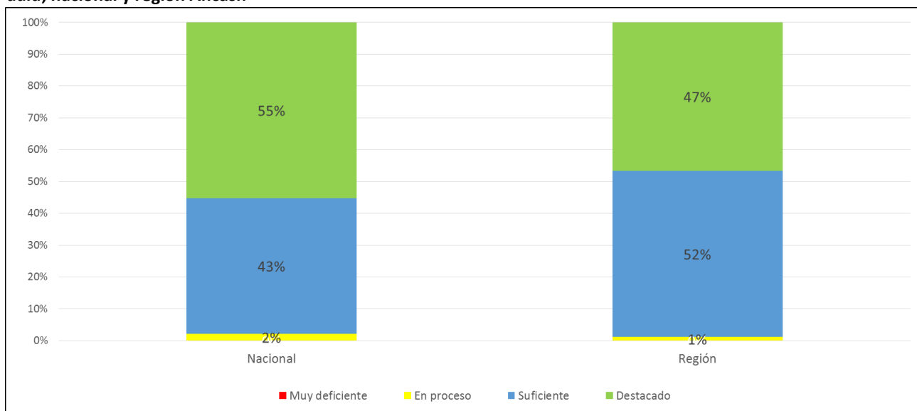
Gráfico 5
